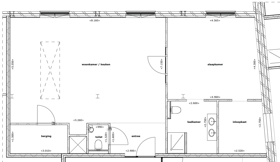
Plattegrond verdieping 03 1:50
